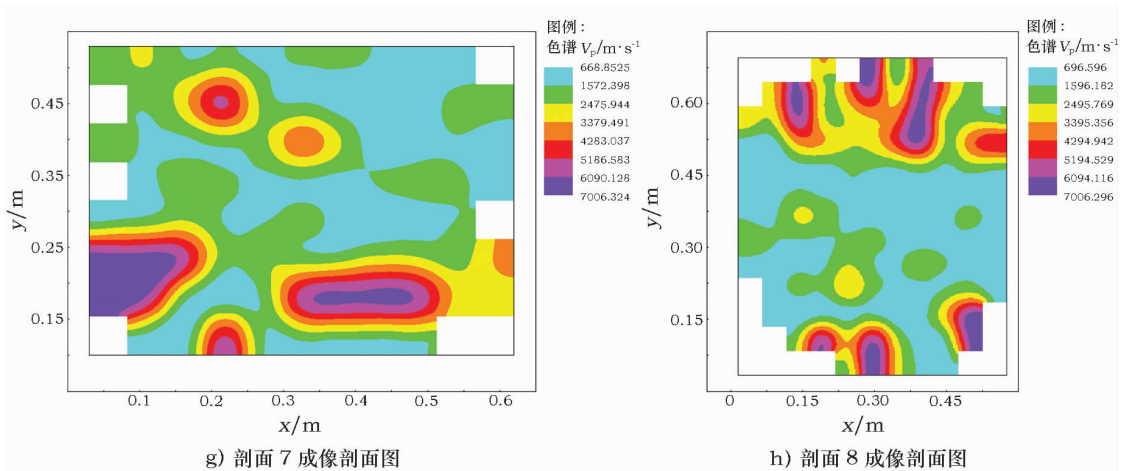
图 6 乾陵西 4 翁仲超声 CT 成像剖面图
