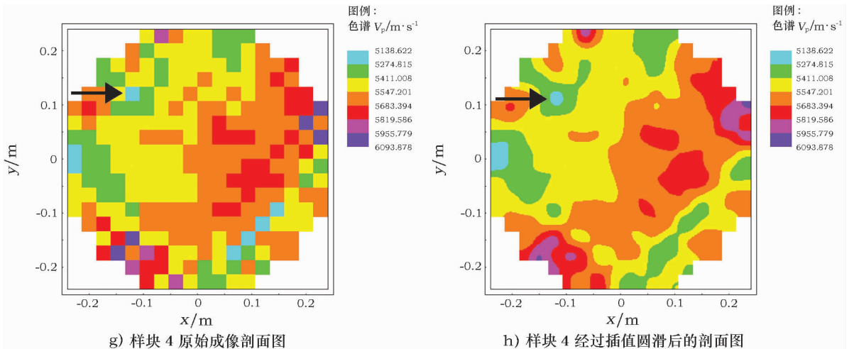
图4 标准样块成像剖面
