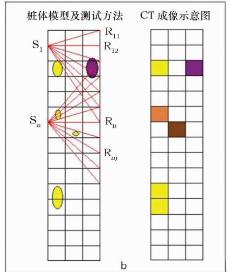
图 2 超声波 CT 成像原理图
