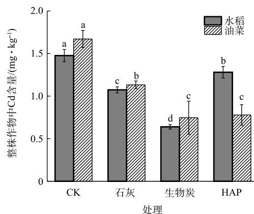
图4 3种处理后整株作物中Cd的含量
