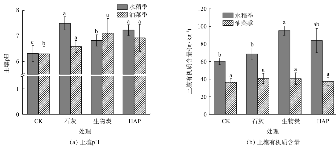
图2 3种处理后土壤pH及有机质含量的变化
