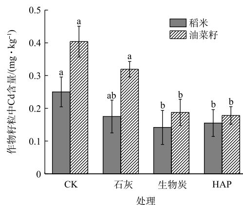
图5 3种处理后作物籽粒中Cd含量
