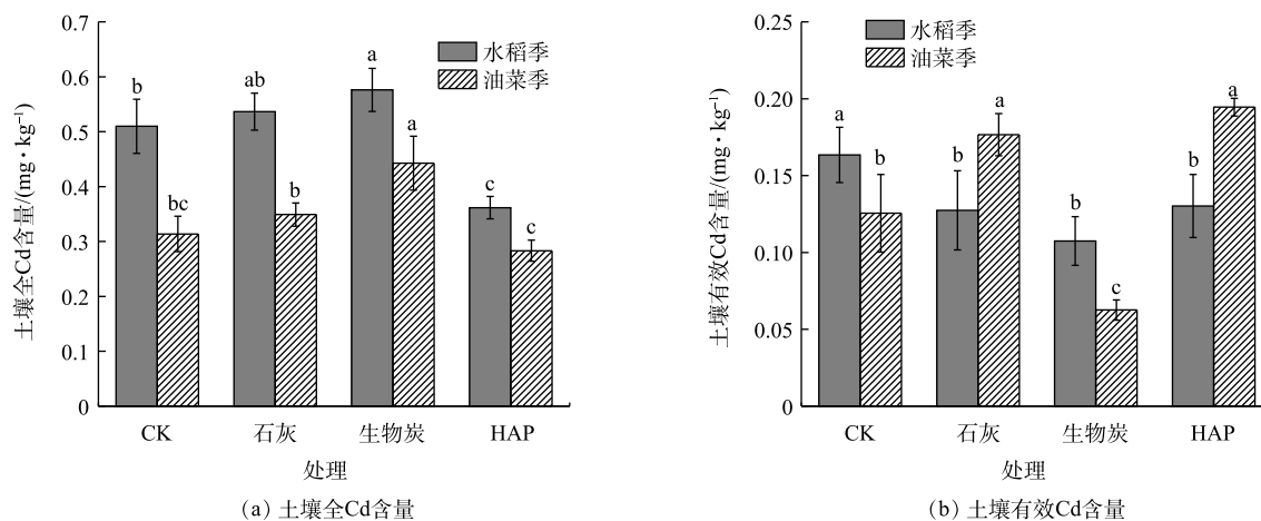
图3 3种处理对土壤Cd含量的影响
