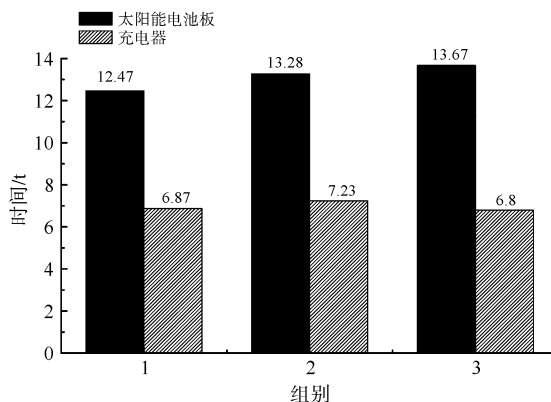
图 7 服装上蓄电池充电时间测试结果
