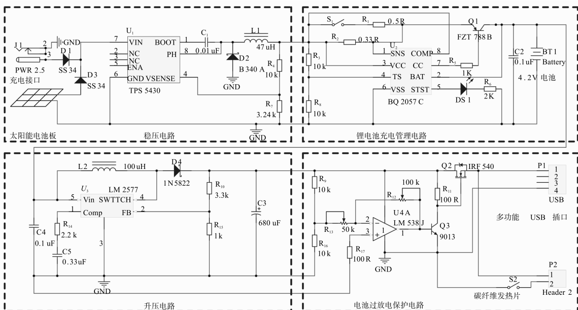
图 4 电路设计
