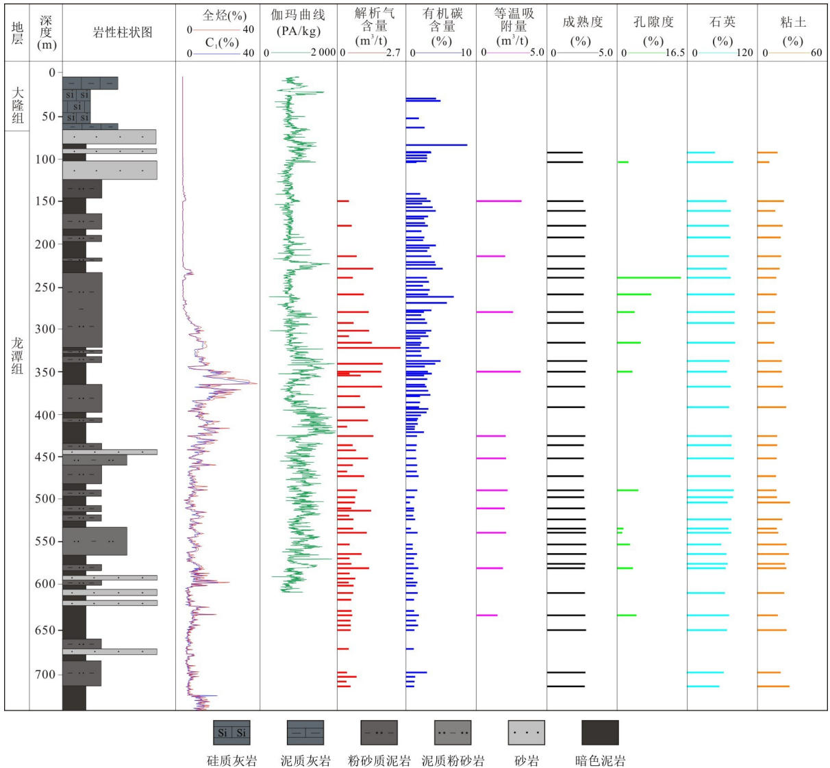
图 3 页岩气调查井 2015H-D3 井龙潭组综合柱状图
