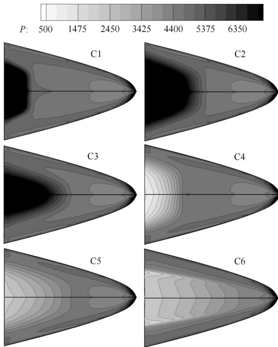
图 13 不同压缩面乘波体压力分布比较
