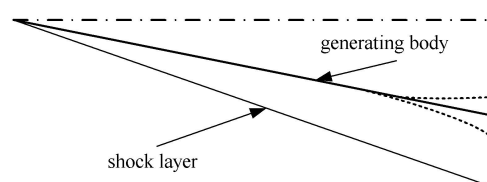
图 2 具有相同激波面的源几何体
