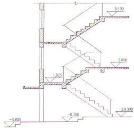
第 8 题图 楼梯局部剖面
