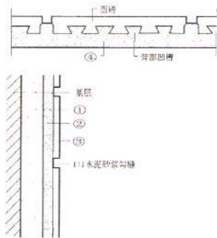
第 7 题图 陶瓷面砖饰面构造示意
