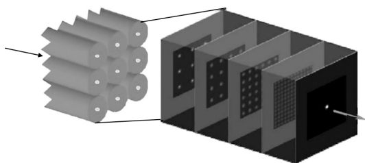
图 20 自成像波导 9 路相干光束合成示意图
