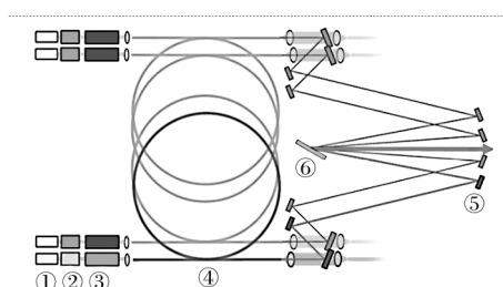
图 9 4 路 MLDG 光谱合成实验结构
