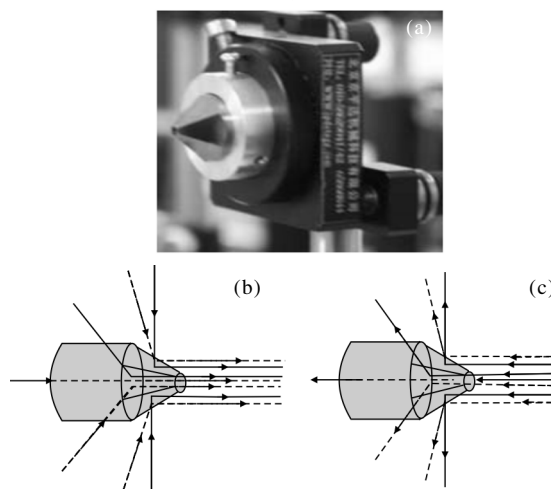
图 15 (a) 六棱台, (b) 六棱台合束, (c) 六棱台分束
