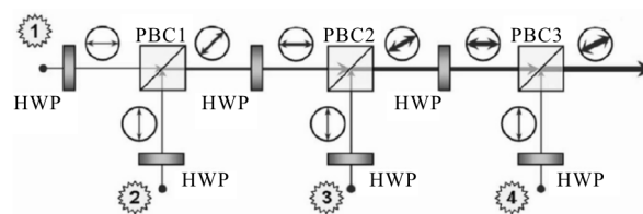
图 22 相干偏振合成示意图
