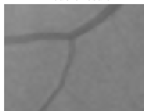
SI-3 result
