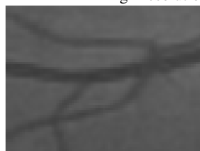
Bicubic result
