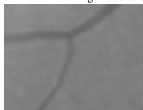
Bicubic result
