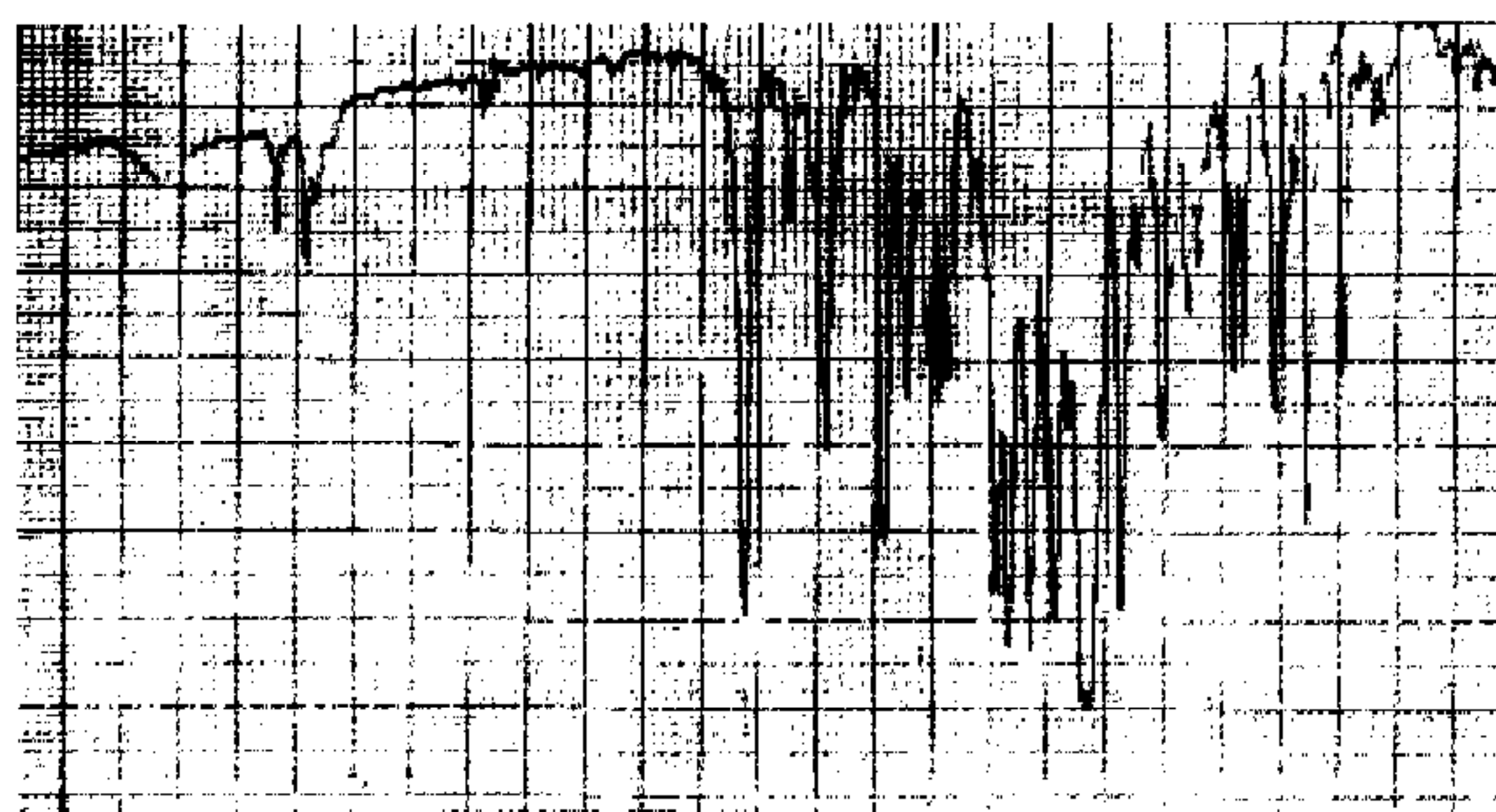
图 1 高效氯氟氰菊酯的标准红外光谱图
