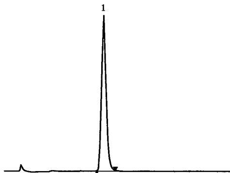
图 3 乙羧氟草醚原药的高效液相色谱图
