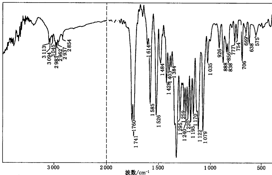
图 1 乙羧氟草醚标样的红外光谱图
