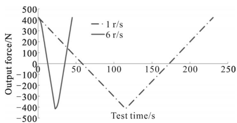
图 3 力促动器输出力范围
