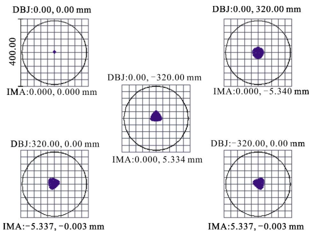
图 8 系统的点斑图
