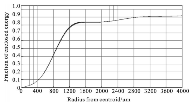
图 10 系统衍射能量集中度曲线
