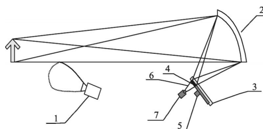
图 5 系统结构图
