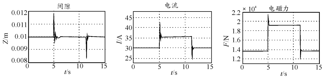
图 4 方案 A 竖曲线段运行情况 (速度 60 km/h, 半径 1 500 m, 坡度 70‰)
