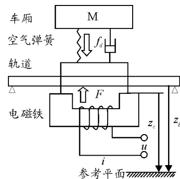
图 1 单点磁悬浮控制模型
