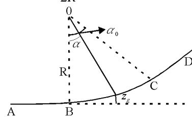
图 3 轨道竖曲线结构示意图
