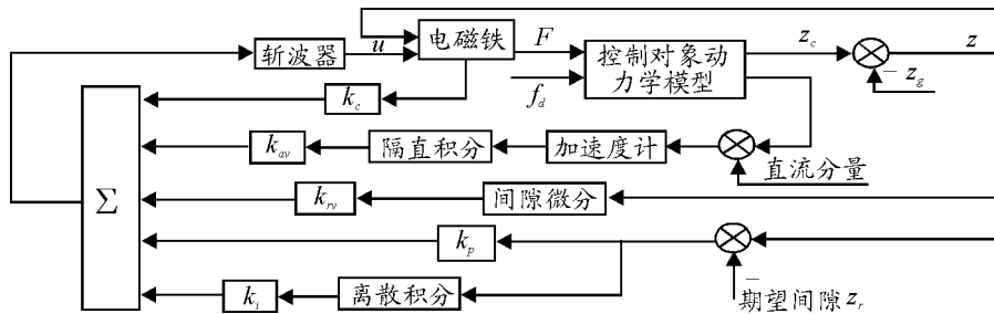
图 2 A 控制方案结构框图
