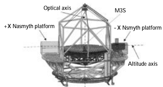
图 1 TMT 简图
