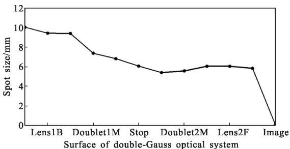
图 2 激光束在各镜面上的光斑尺寸
