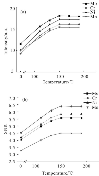
图 3 不同样品温度条件下的光谱强度和信噪比
