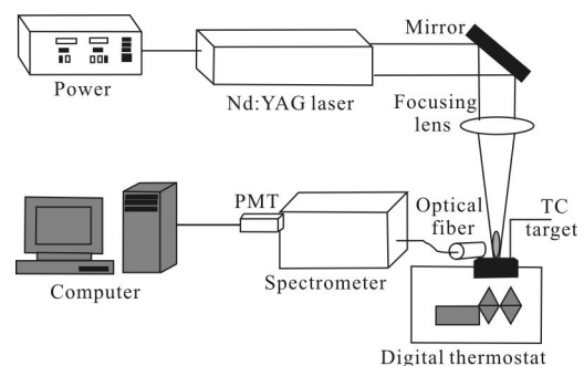
图 1 LIBS 实验装置示意图
