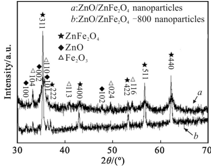
图 2 未退火、退火后的 ZnO/ZnFe 2 O 4 复合纳米粒子的 XRD Fig.2 XRD patterns of the synthesized and annealed ZnO/ZnFe 2 O 4 nanoparticles
