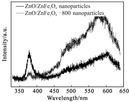
图 3 未退火和退火后的 ZnO/ZnFe 2 O 4 复合纳米粒子的 PL Fig.3 PL spectroscopy of the synthesized and annealed ZnO/ZnFe 2 O 4 nanoparticles
