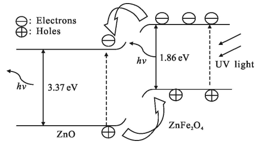
图 4 ZnO/ZnFe 2 O 4 II 型能带结构示意图 Fig.4 Type-II energy band structure of ZnO/ZnFe 2 O 4 nanocomposites schematic diagram
