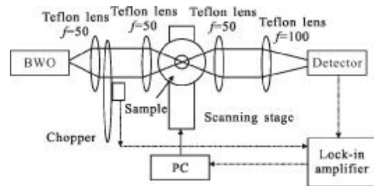
图 1 THz-CT 实验平台
