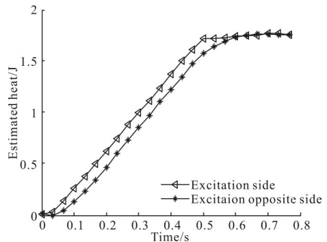
图 5 裂纹生热估计
