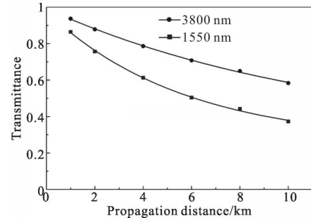
图 10 能见度为 10 km 的光子数随距离变化的曲线
