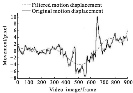
(b) 垂直方向位移
