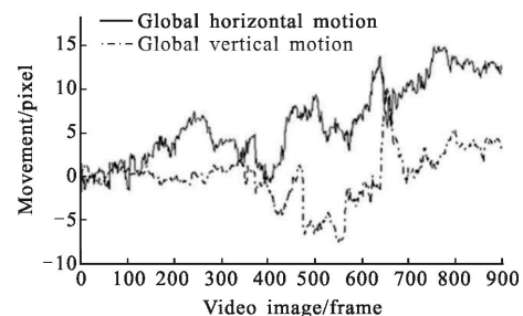
图 3 全局平移运动参量曲线
