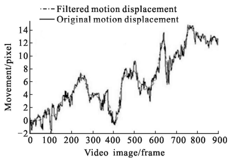
(a) 水平方向位移
