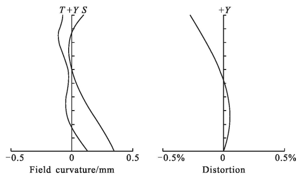
图 4 场曲和畸变曲线图
