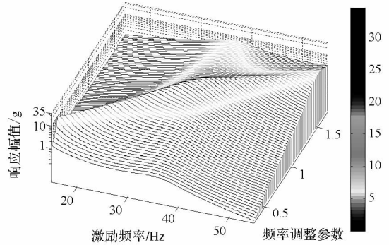
(a) 响应曲线 - 侧视
