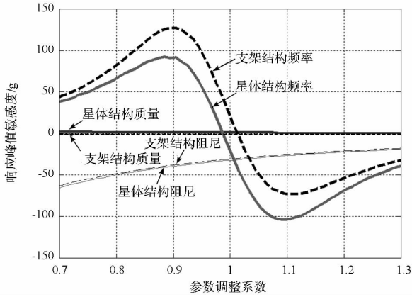
图 9 响应峰值相对各参数调整系数的敏感度曲线
