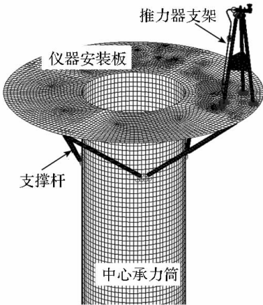
图 2 星架系统的有限元模型
