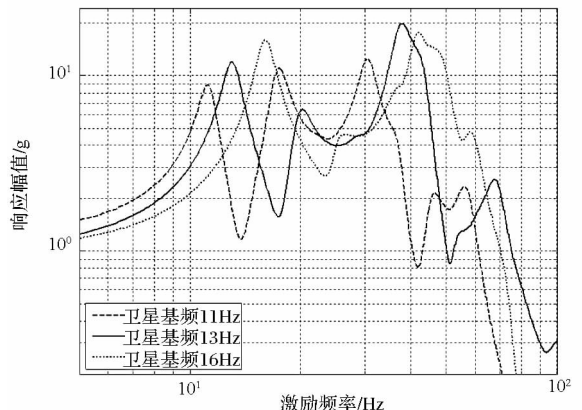
(a) 推力器激励方向频率响应曲线
