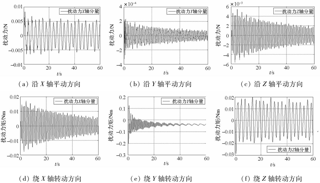
图 8 含质心偏置工况扰动力/力矩时间历程
