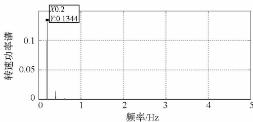
(b) 转速功率谱
