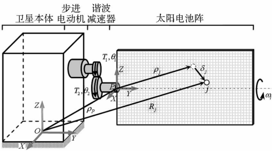
图 1 电池阵结构示意图
