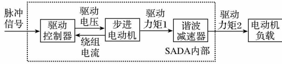
图2 SADA 驱动环节
