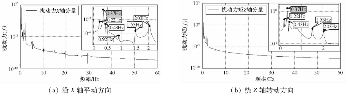
图 9 含质心偏置工况扰动力/力矩频谱曲线
