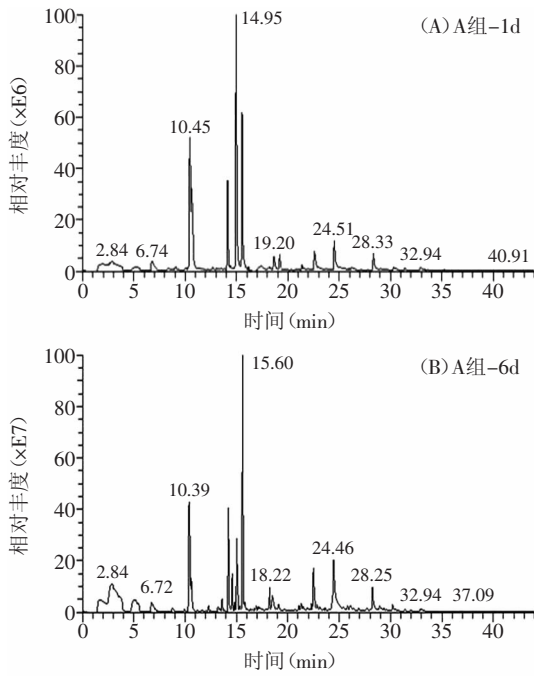
图1 A组线椒香气成分GC-MS总离子图
