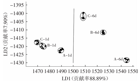
图6 贮藏后货架3个处理组的线性判别分析
