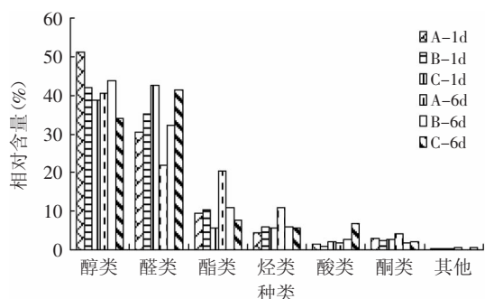
图4 贮藏后货架线椒挥发性物质种类相对含量的变化
