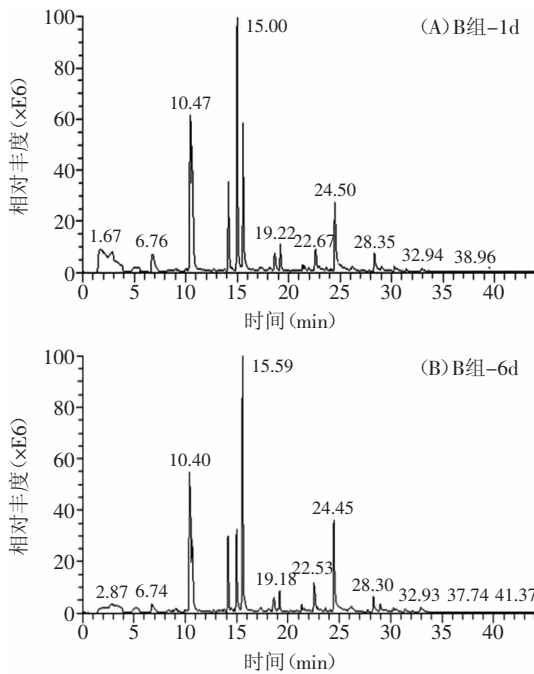
图2 B组线椒香气成分GC-MS总离子图
