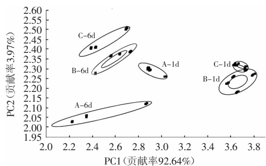
图5 贮藏后货架3个处理组的主成分分析
