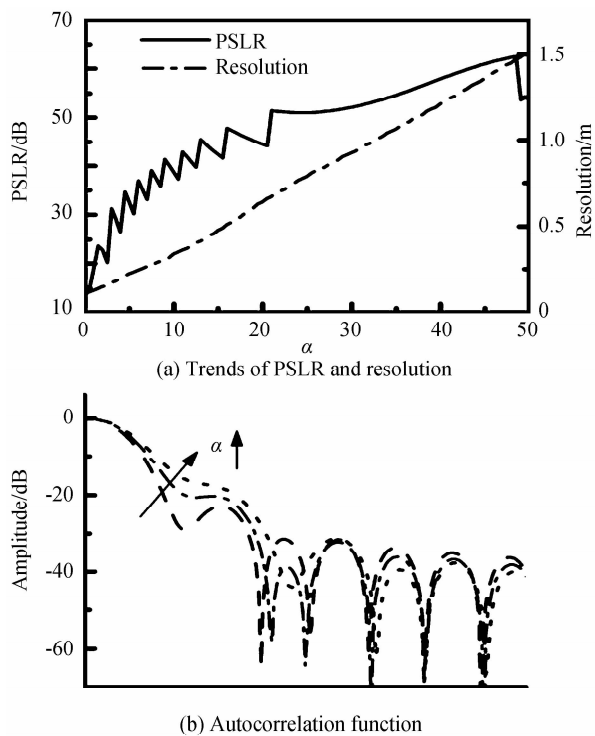
图 5 PSLR 和空间分辨率
