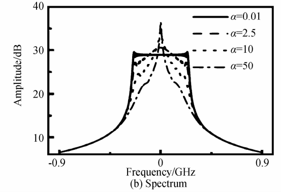
图 3 不同 \alpha 值非线性调频脉冲信号
