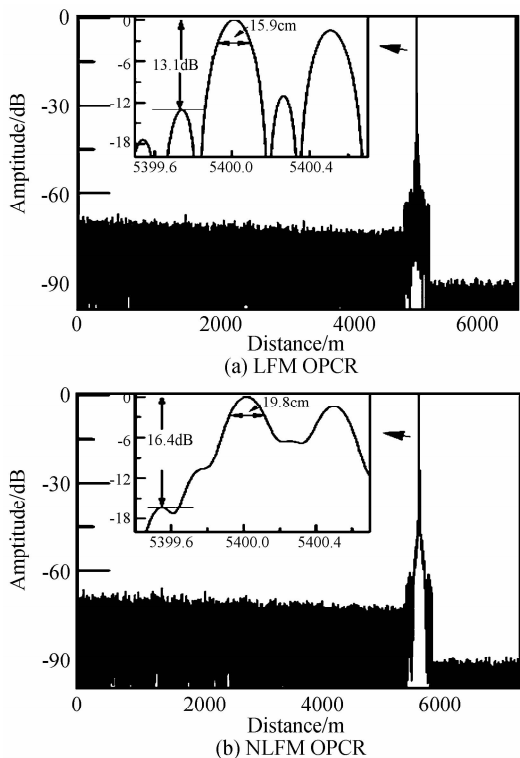
图 6 不同频率调制方式下的 OPCR 系统仿真结果对比
