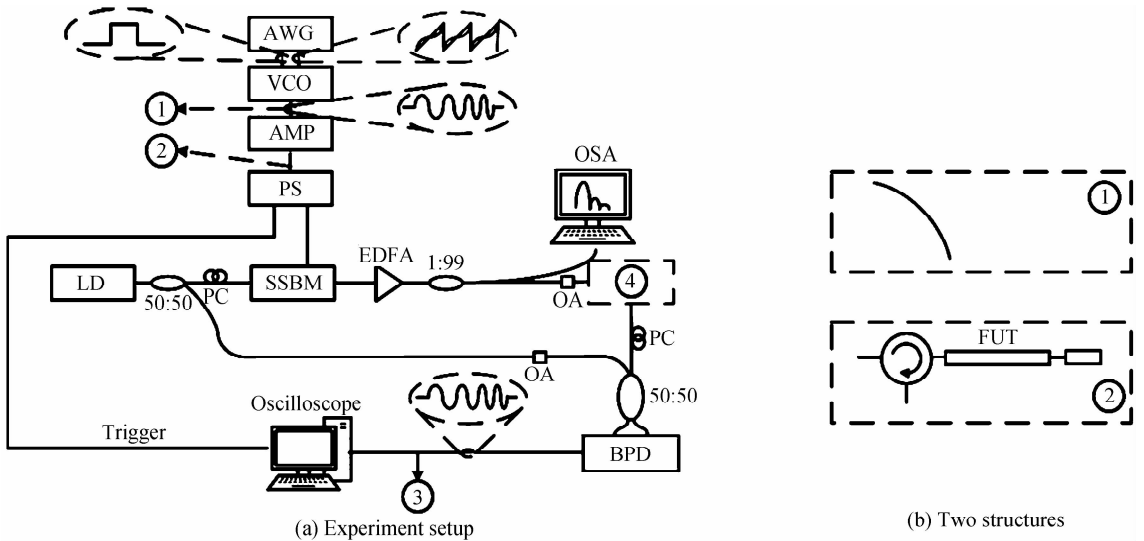
图 7 OPCR 实验系统图 Fig. 7 Experiment setup of OPCR system
