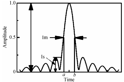
图 2 自相关函数空间分辨率和 PSRL 的定义
