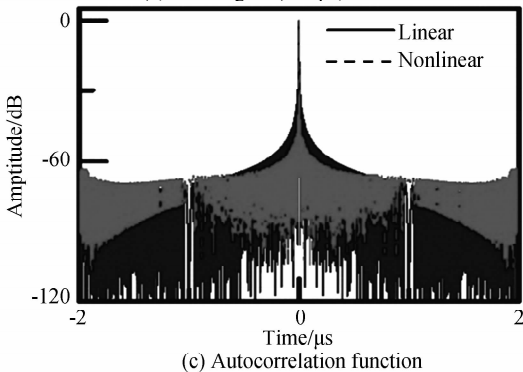
图 4 调频脉冲信号及其自相关函数
