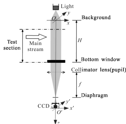
图 4 气动光学波前测量装置光路示意图
