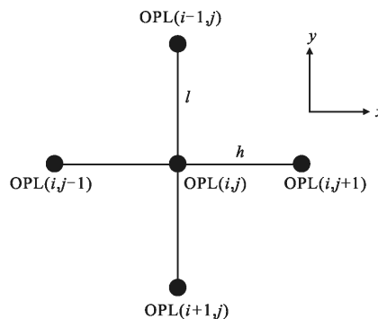
图 3 Southwell 算法积分网格示意图
