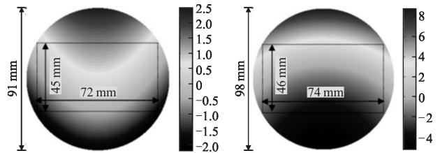
(b) 第一片反射镜面型
