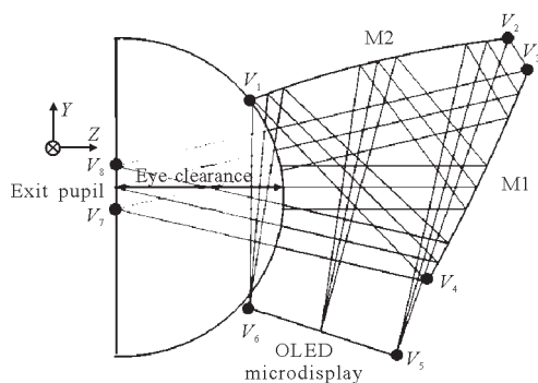
图 2 双反射镜 HMD 光路图
