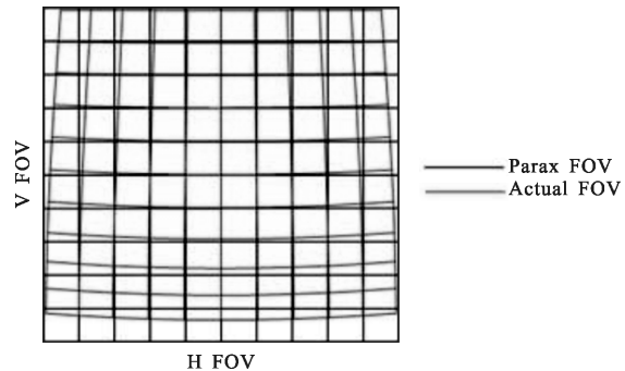
图 7 HMD 的畸变
