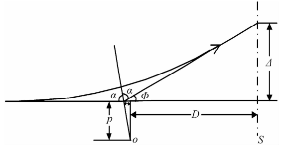
图 4 偏折角和偏折位移量关系图 Fig. 4 The deflection angle corresponding to fringe shift 各角度关系为
