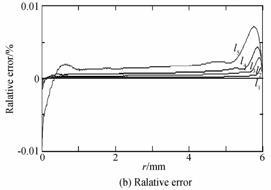
图8 折射率反演值和相对误差
