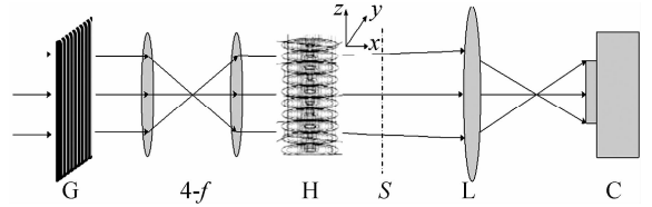
图1 编码源成像光路设计原理
