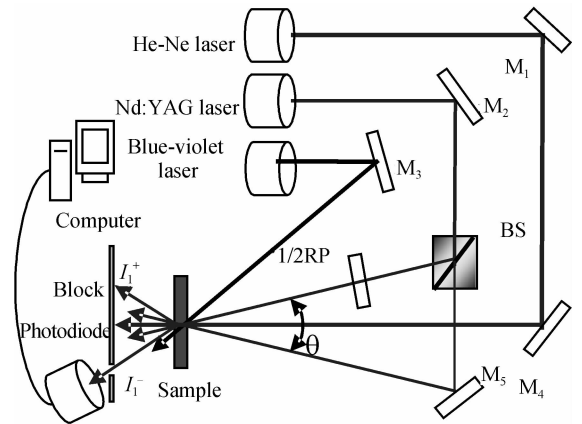
图 3 螺吡喃掺杂聚合物薄膜偏振全息记录实验装置 (BS 表示分光镜; M_1 - M_5 为反射镜; 1/2RP 为 1/2 相位延迟片)
