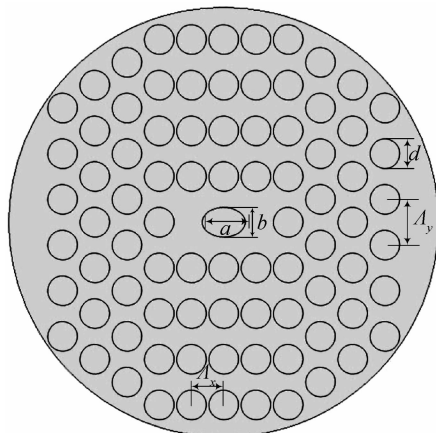
图1 双芯光子晶体光纤截面图
