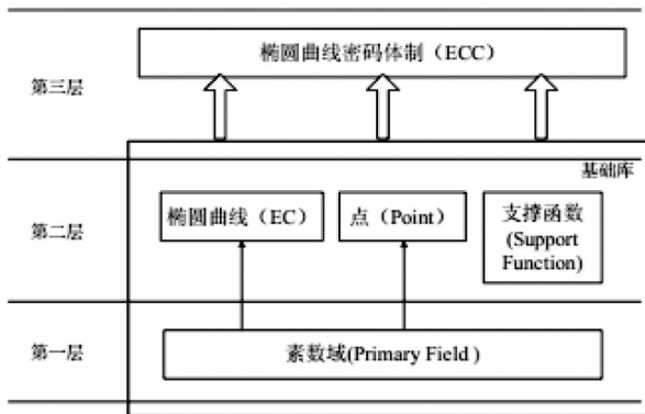
图 3 ECC 模块层次结构
