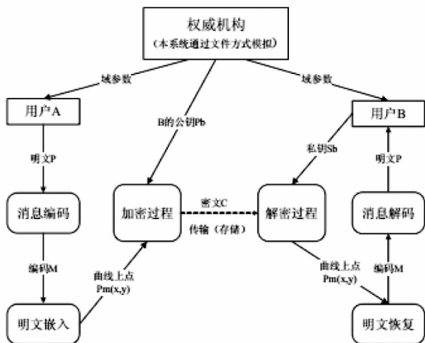
图 4 加密 / 解密数据流
