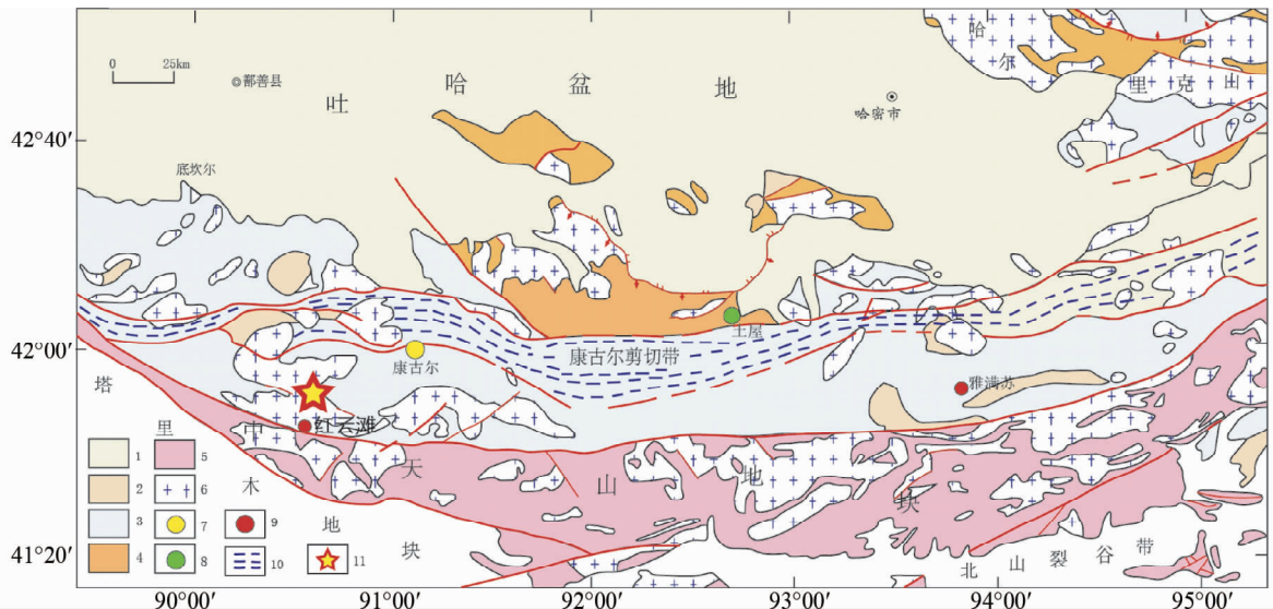
图1 东天山构造格架地质简图(据王京彬等, 2006 修改)
