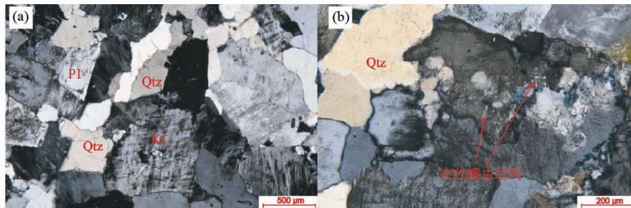
图2 红云滩岩体花岗闪长岩显微照片
