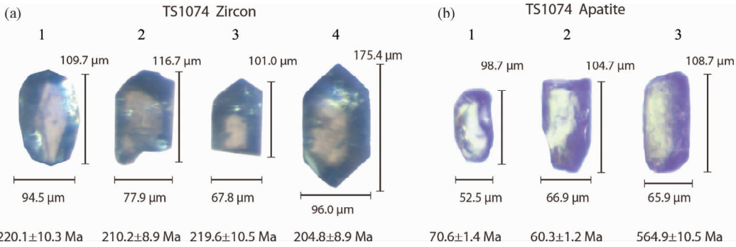
图 5 红云滩花岗岩闪长岩锆石 (a) 和磷灰石 (b) 显微照片
