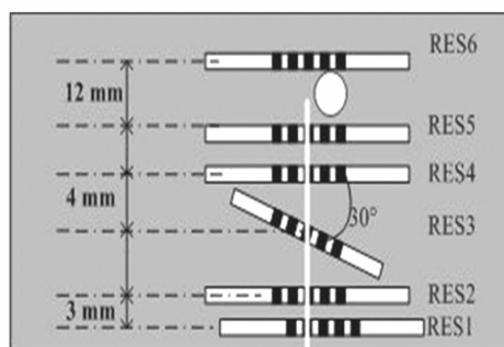
图 2 静态加载实验系统图
