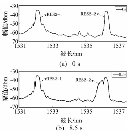
图8 动态加载实验 RES2-1 与 RES2-2 光谱结构图
