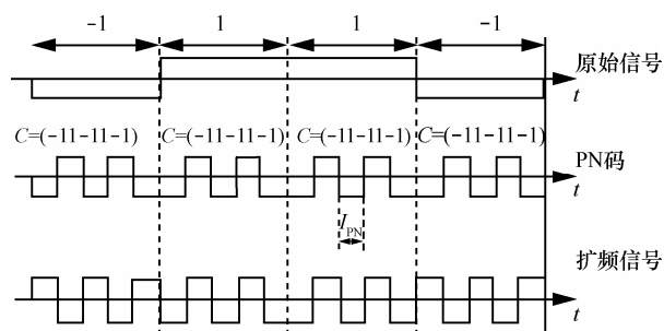
图 5 DSSS 原理
