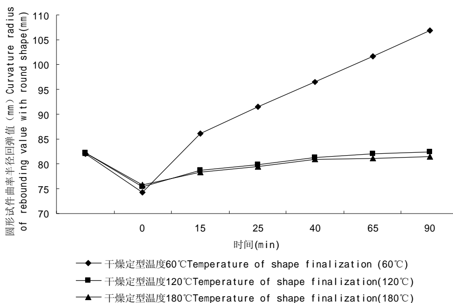
图5 圆形试件回弹曲线
