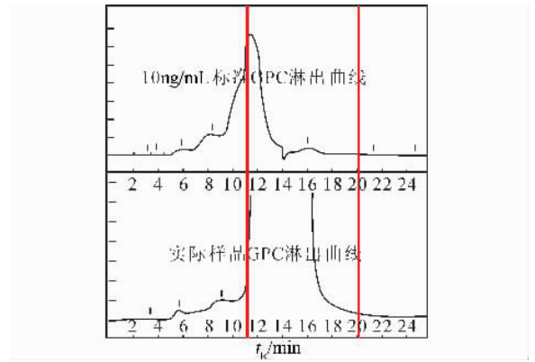
图 2 标准品及实际样品的 GPC 淋洗曲线
