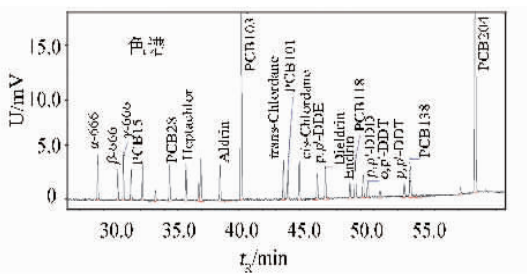
图 1 22 种化合物的 GC-ECD 色谱图
