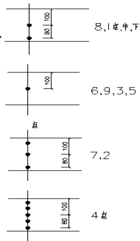
测温点竖向布置图
