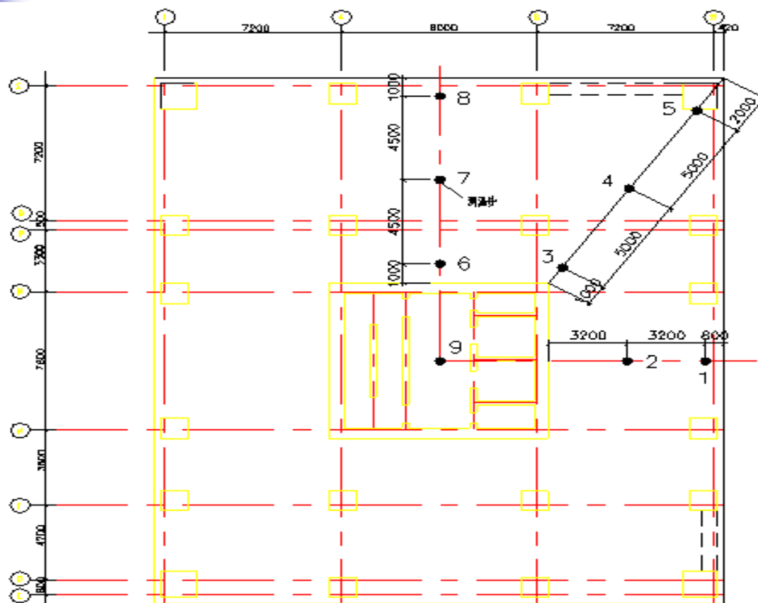
测温点平面布置图
