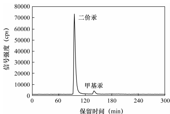
图4 乳粉样品中汞形态的色谱分离图
