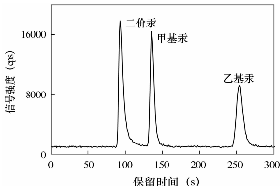
图3 IC-ICP-MS 联机检测汞的各种形态的分离色谱图(浓度以汞计均为 10 \mu\text{g/L} )
