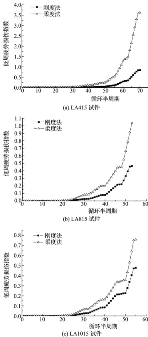
图2 纵筋低周疲劳损伤指数
