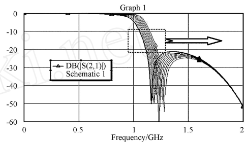
(b) 低通原型滤波器的频率响应,可见其三个传输零点,其中第一传输零点为 1.22 GHz
