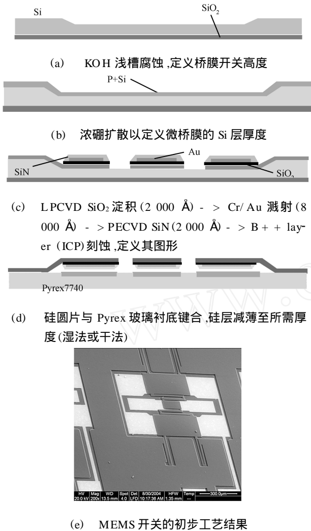
图 4 MEMS 桥膜开关的体硅工艺加工工艺流程及开关流片结果
