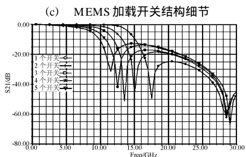
(d) 分别加载 1-5 个开关后滤波器的响应 图 3 基于体硅加工的微机械开关的 7 阶可调节椭圆低通滤波器设计及其滤波特性的全波分析结果
