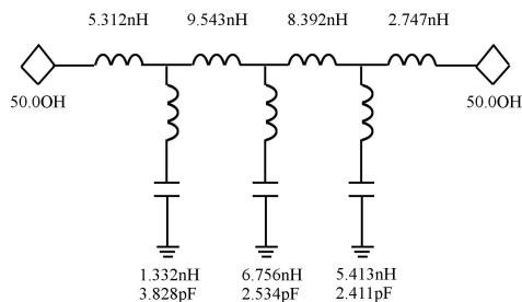
(a) 7 阶椭圆低通滤波器原型电路
