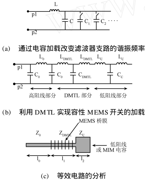
图 2 基于 DMTL 的滤波器滤波特性调节方法
