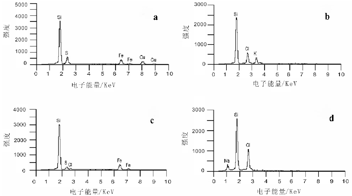
图3 流体包裹体中子矿物的能谱图
