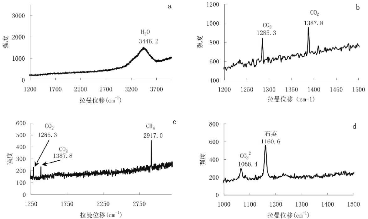
图4 流体包裹体气液相成分的LRM谱图
