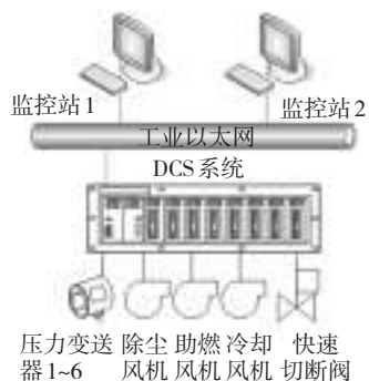
图1 煤气安全控制系统
