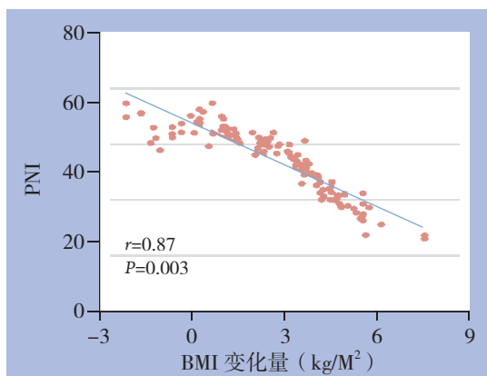
图 1 老年胃癌患者 BMI 变化量与 PNI 的相关性
