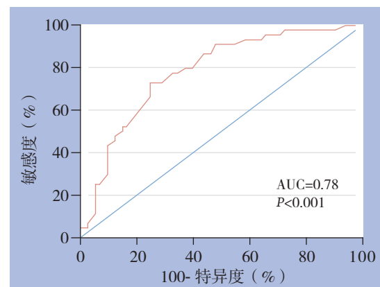
图 2 BMI 变化量预测老年胃癌患者预后的 ROC 曲线
