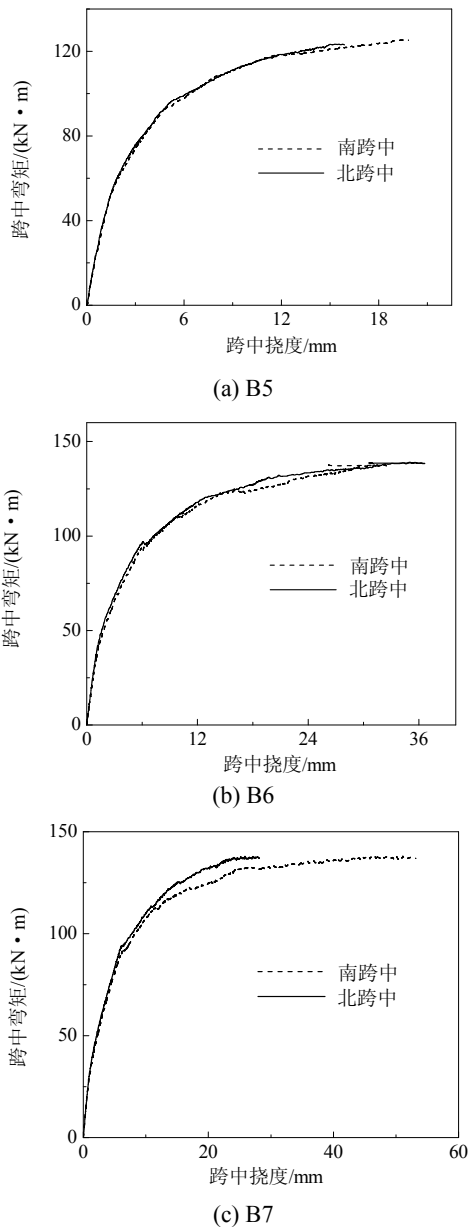
图 4 试验梁的荷载-挠度曲线
