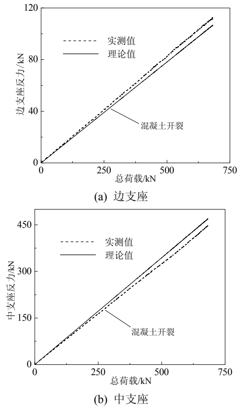
图 5 B7 梁的荷载-支座反力曲线
