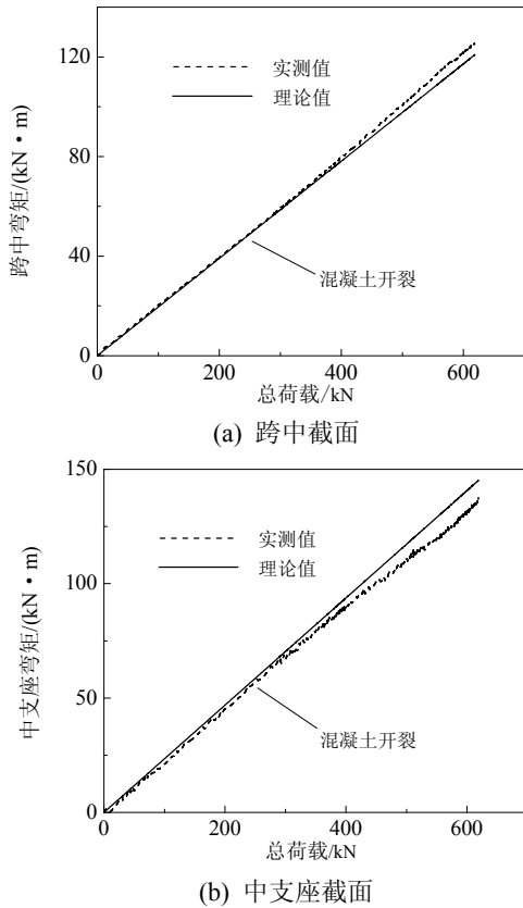
图 6 B5 梁的截面弯矩-荷载曲线 Fig.6 Load-flexural moment curve in specimen B5
