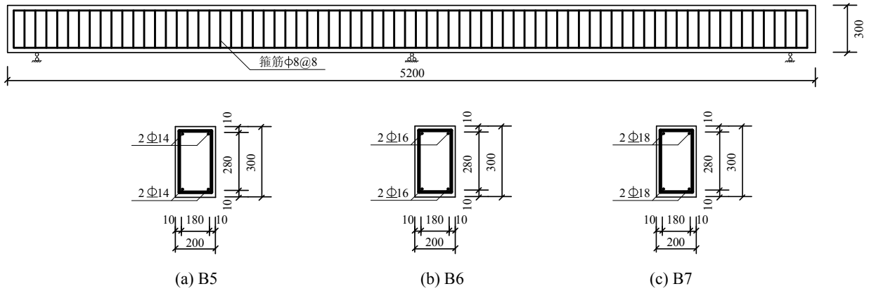
图2 试验梁截面尺寸及配筋 /mm
