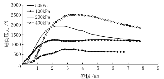
(b) 饱和原状土三轴试验应力-应变曲线
