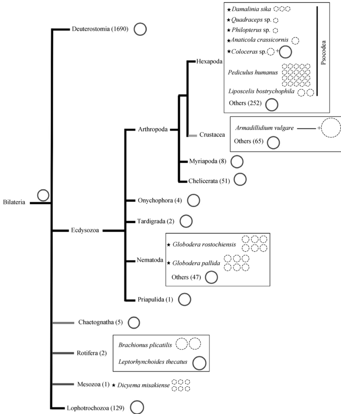
图 2 2627 种两侧对称动物线粒体染色体的结构图 [15]
