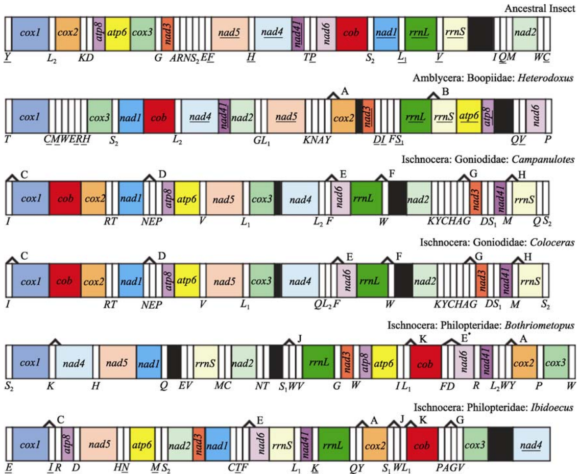
图 3 虱目线粒体基因组的完整基因组 [14]
