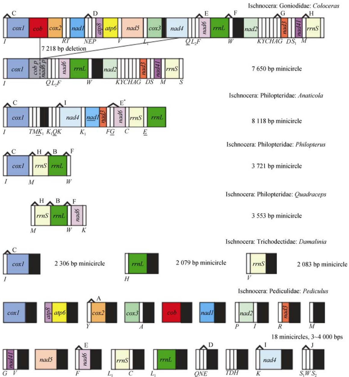
图 4 虱目微环线粒体基因组的基因图 [14]
