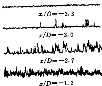
图6 典型壁面信号
