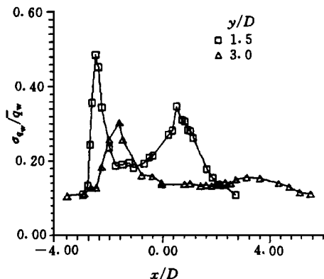
图 10 干扰区非中心线上热流率脉动无量纲标准偏差( A = 0^\circ )
