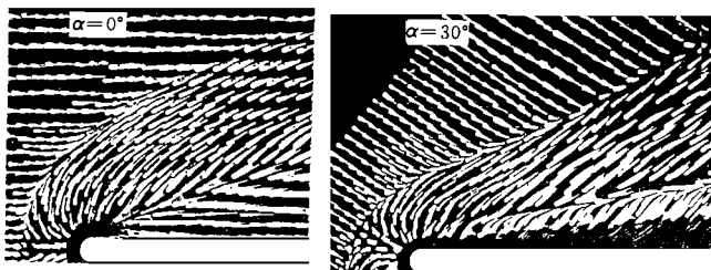
图 2 油流流谱图
