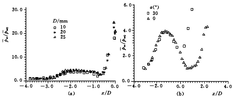
图 8 平板干扰区平均压力 (a)中心线上;(b)非中心线上( y/D = 1.75 )
