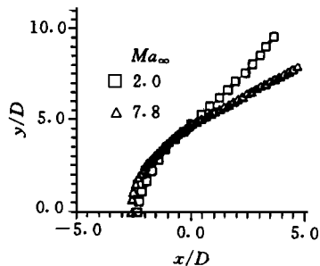
图 3 Mach 数对主分离线的影响
