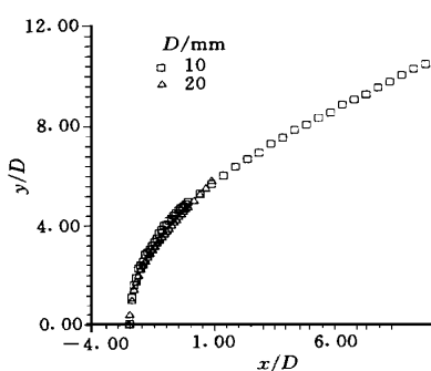
图4 前缘直径对主分离线的影响
