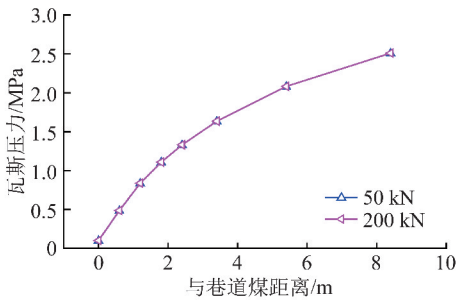
图9 煤层瓦斯流动规律和分布特征
