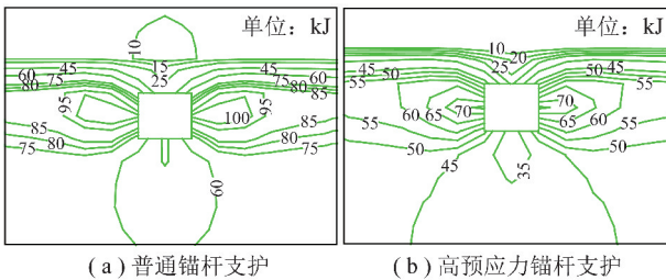
图3 巷道两帮弹性能分布特征
