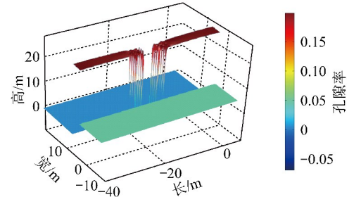
(b) 高预应力锚杆支护
