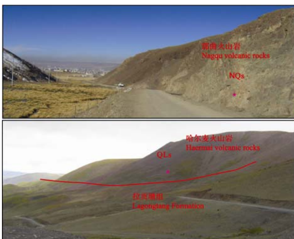
图 3 那曲地区中生代火山岩地貌景观 Fig. 3 Landscape of Mesozoic volcanic rocks in Nagqu area
