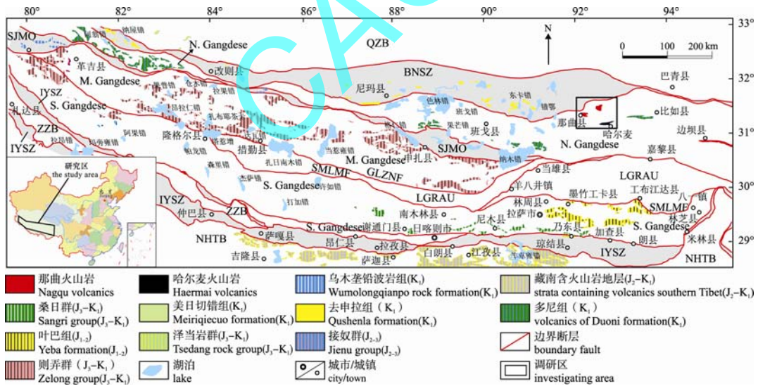
图 1 西藏冈底斯带中生代含火山岩地层分布图
